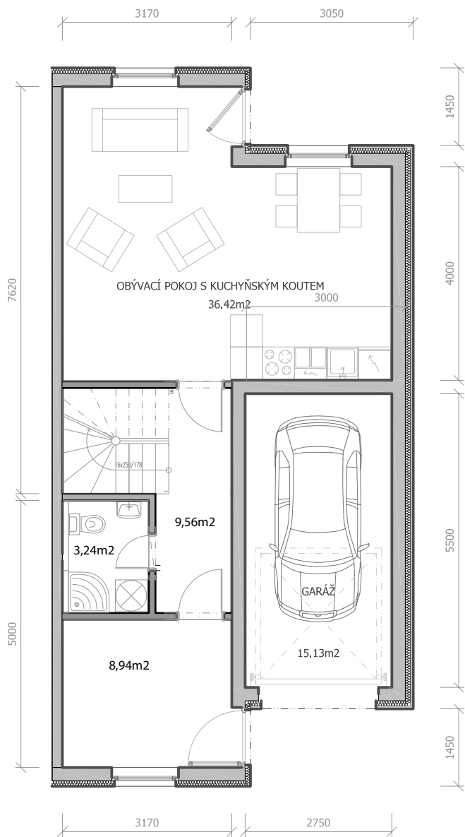
PŘÍZEMÍ
